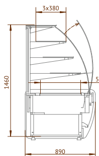
Witryna cukiernicza neutralna
