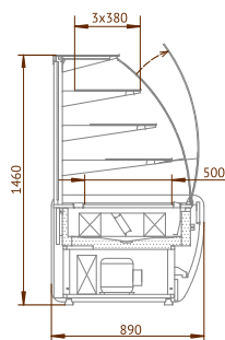
Witryna cukiernicza chłodnicza
